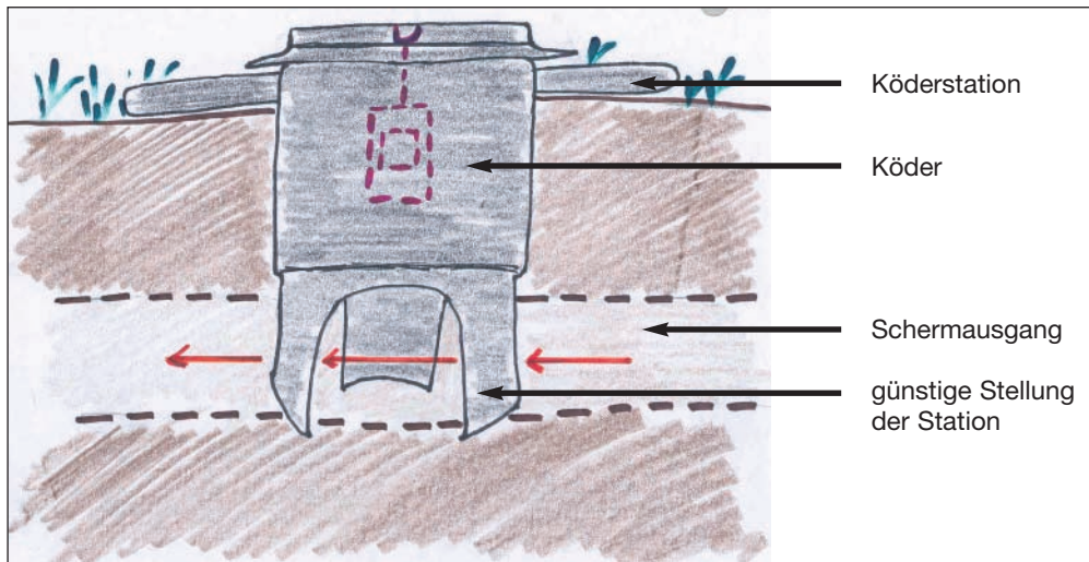
Abb. 11: Eingebaute Köderstation
