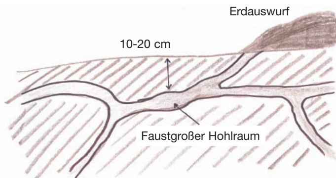
Abb. 10: Einbau von Köderstationen
